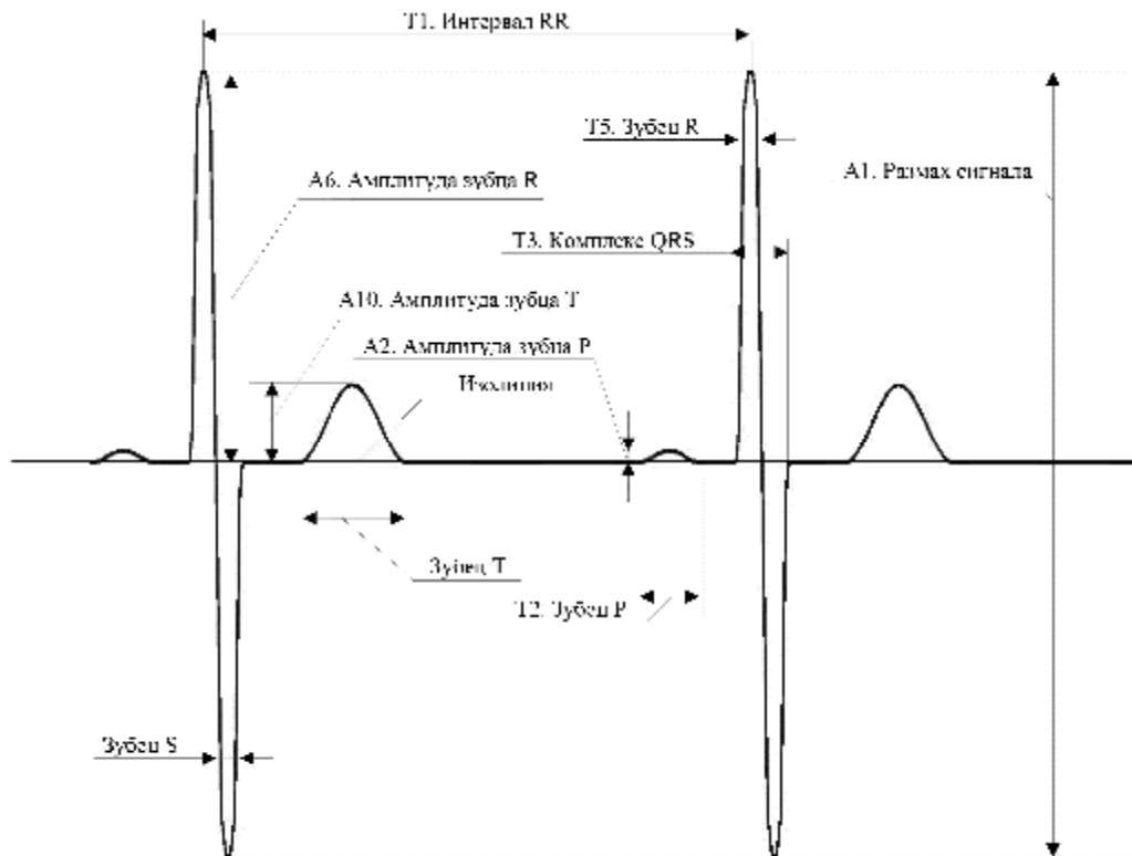
Р и с у н о к В.1 – Форма и наименования амплитудно- временных параметров элементов сигнала «CAL50000»
